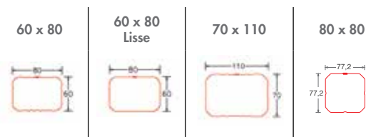
Tuyaux Profilés
